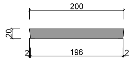
Grille en BFUP
